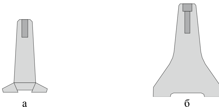
а– высота 50 и 65 см; б– высота 80 см Рисунок 5 –Временные защитные барьеры
