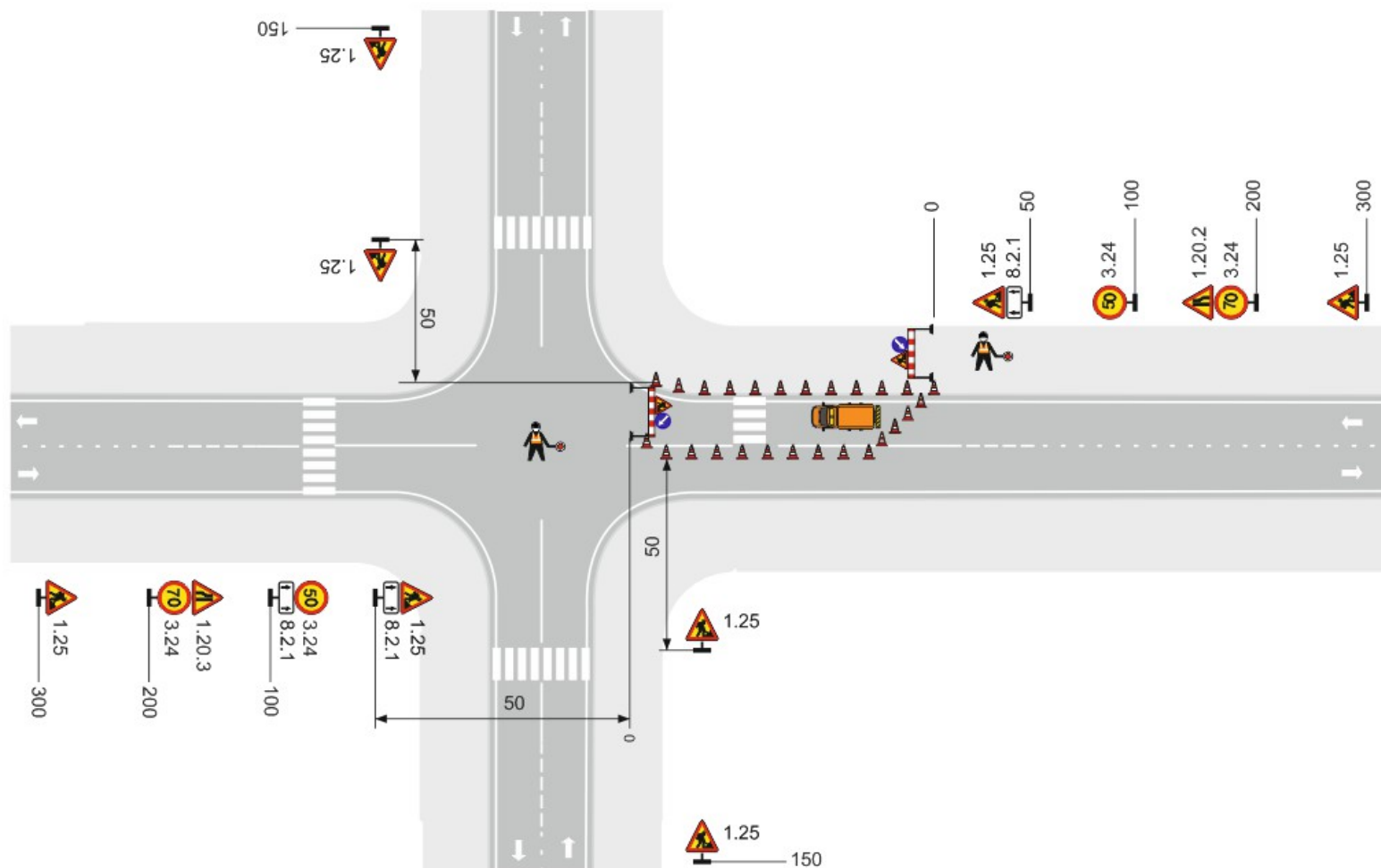
Рисунок Б.39 – Пересечение автомобильных дорог в одном уровне. Рабочая зона производства краткосрочных работ по нанесению дорожной разметки на полосу движения. Пропуск транспортных средств по полосе встречного движения с помощью регулировщиков (при необходимости допускается увеличивать количество регулировщиков)
