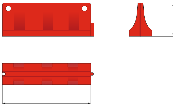
Рисунок 6 – Защитный блок из полимерного материала
